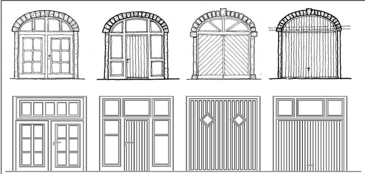
Beispiele für umgebaute Tore mit Korbog oder waagrechtem Sturz.
