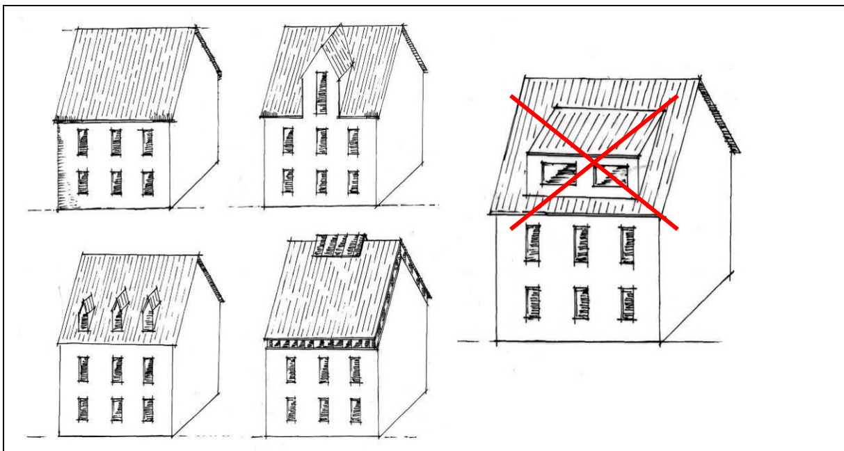
Empfehlenswerte Gaubenformen
