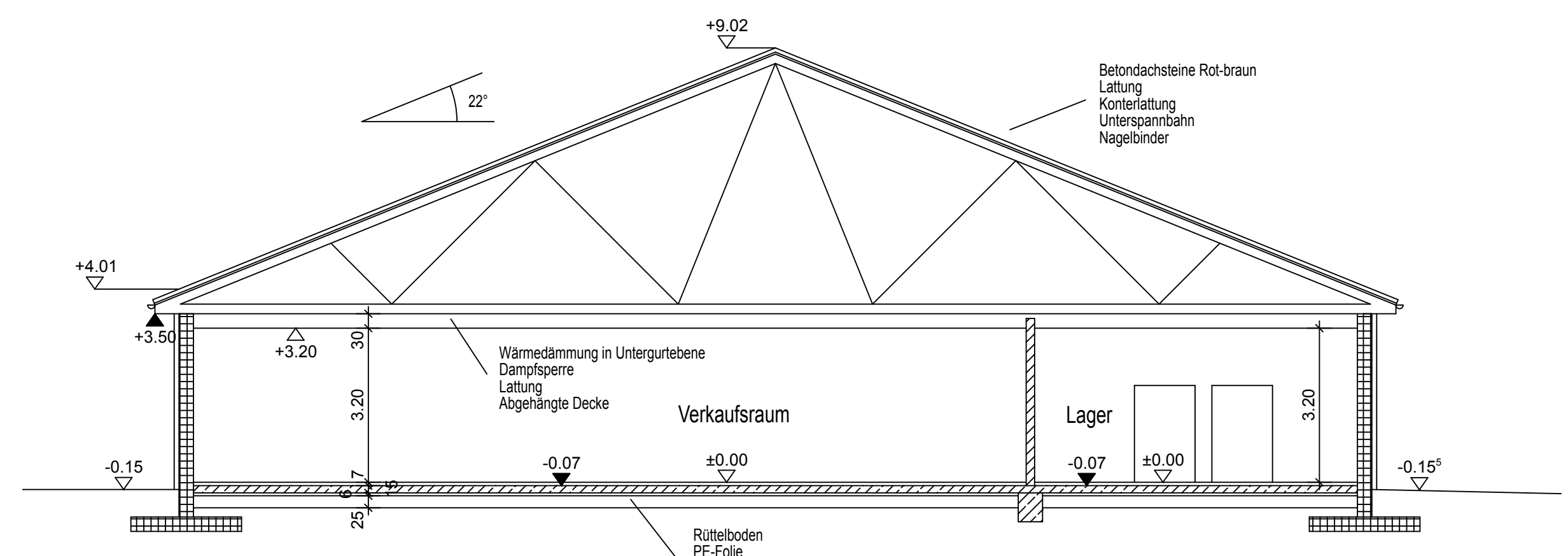
Schnitt A-A
